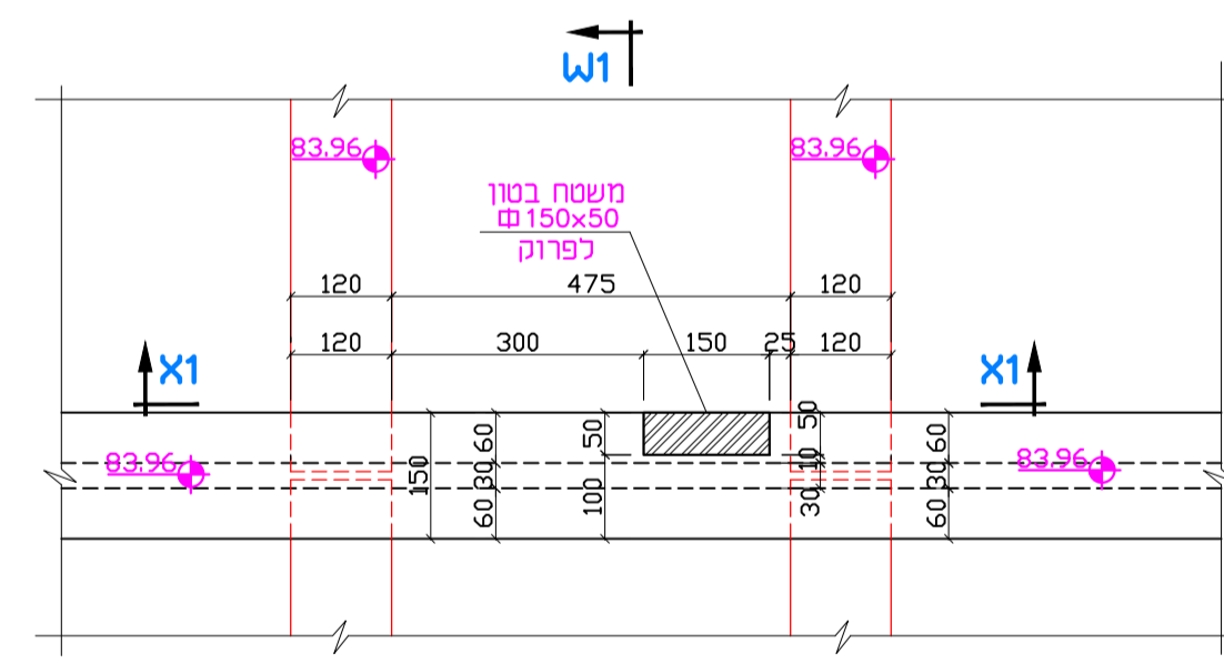
הכנת בטון לפני הנחת פלטת פלדה 1 : 100
