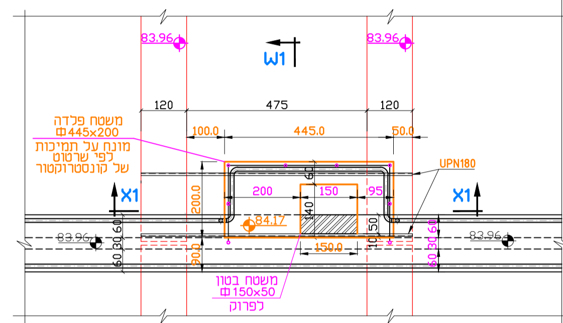
מבט במפלס 83.96 1 : 100
