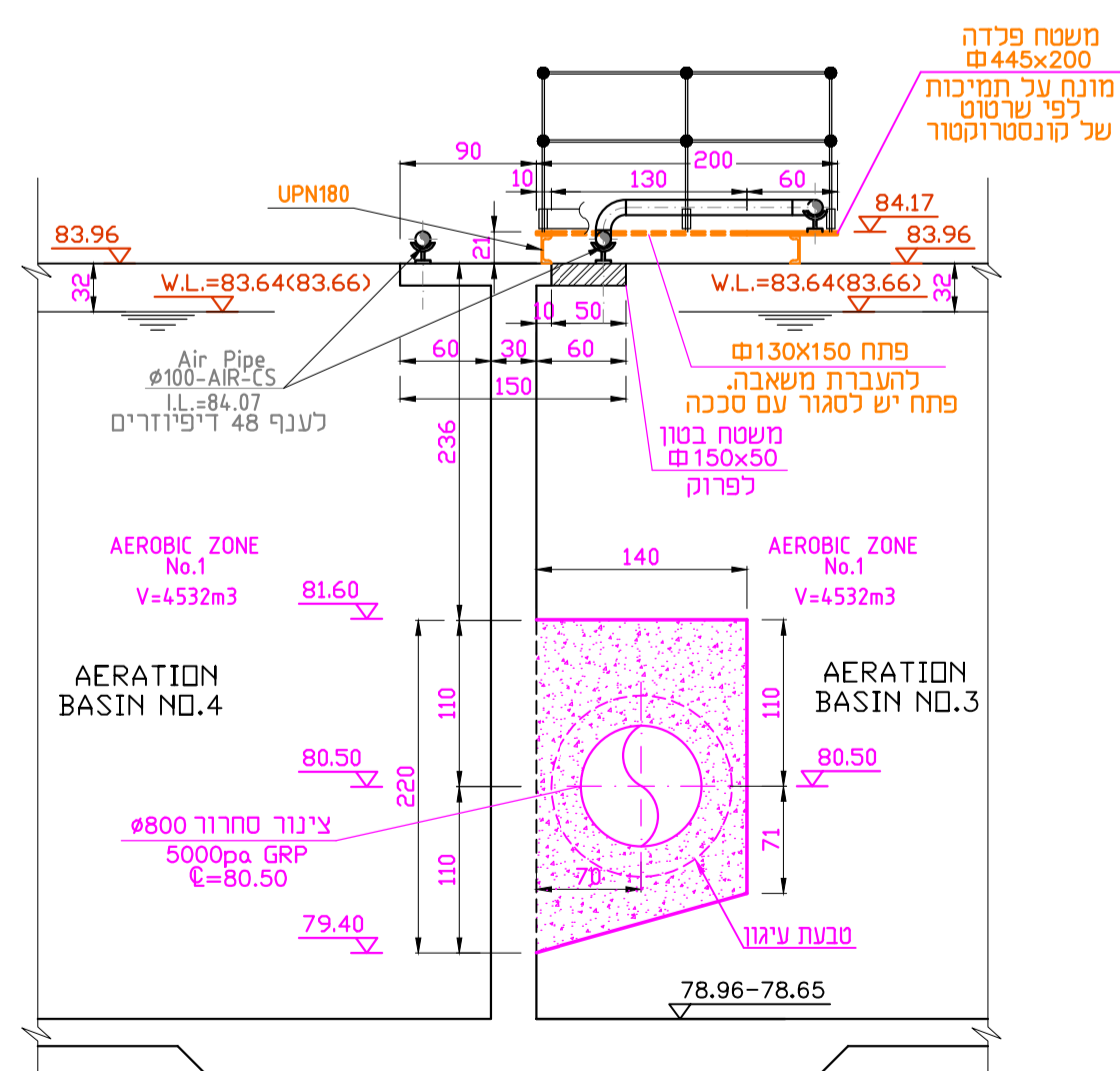
SECTION W1 - W1 1 : 50
