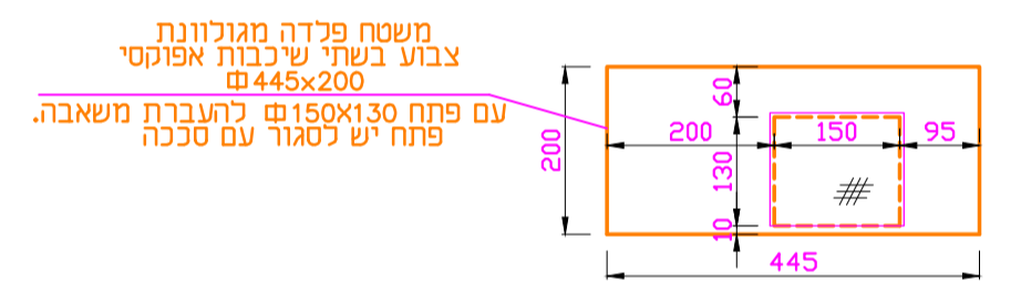
משטח פלדה מגולוונת 1 : 100
